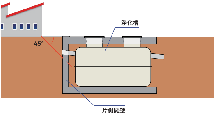
▲片側擁壁のイメージ図
