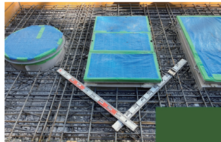
▲マンホール周囲の補強筋の様子
